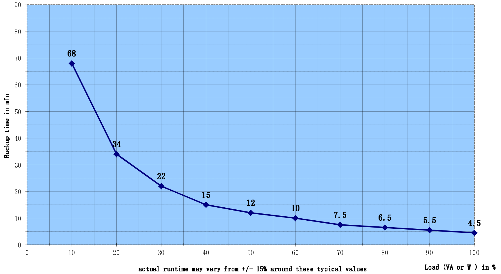
5P 850 for Pf= 0,7 loads (100% = 850 VA / 600 W)
