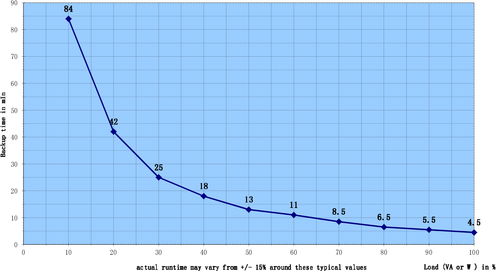
5P 1550 for Pf= 0,7 loads (100% = 1550 VA / 1100 W)
