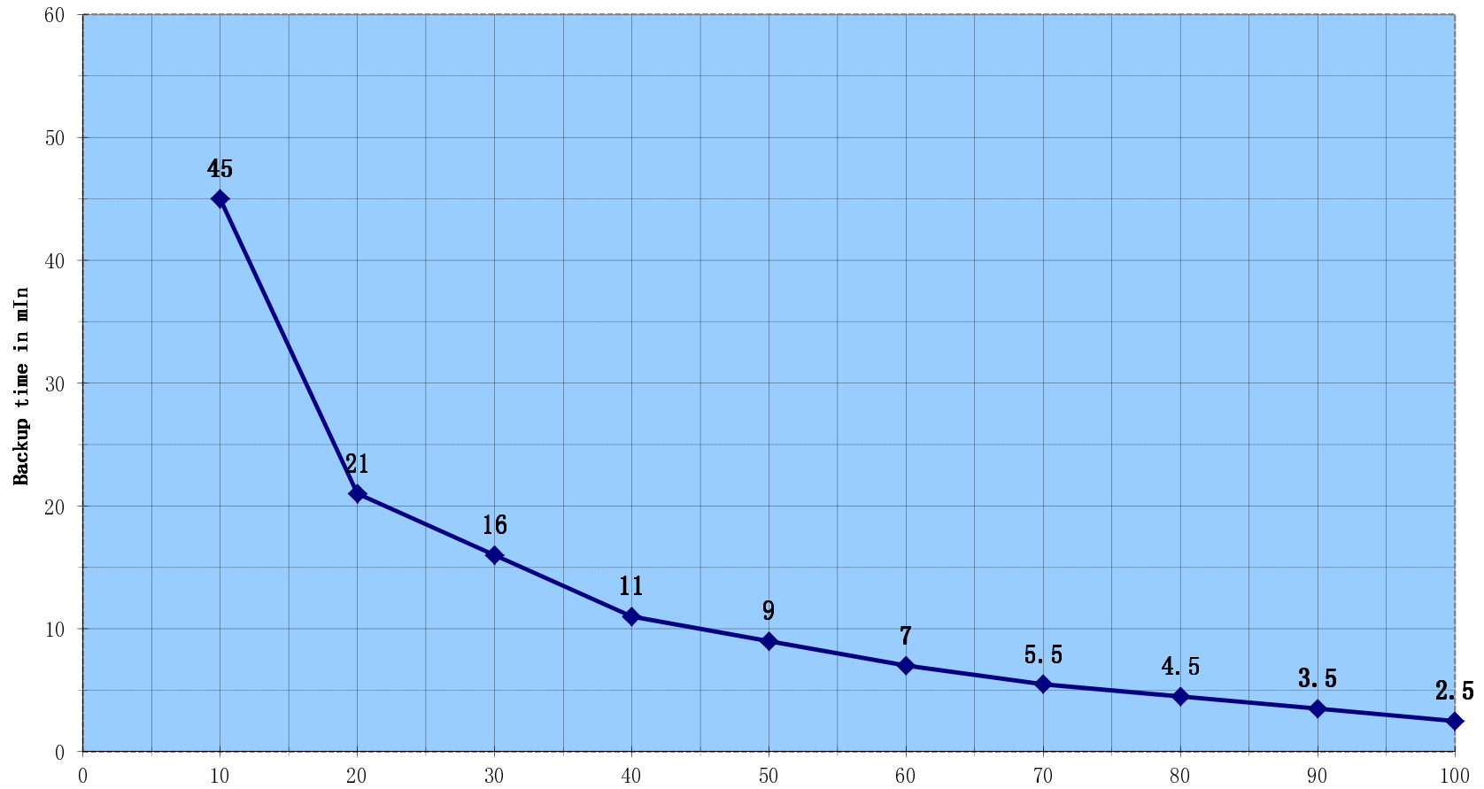
5P 650 for Pf= 0,7 loads (100% = 650 VA / 420 W)
