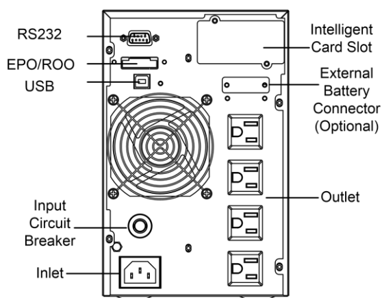
Castle Tower 1K(S)-LV 後面板視圖
