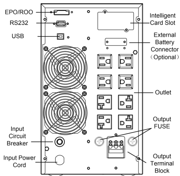
Castle Tower 3K-LV 後面板視圖
