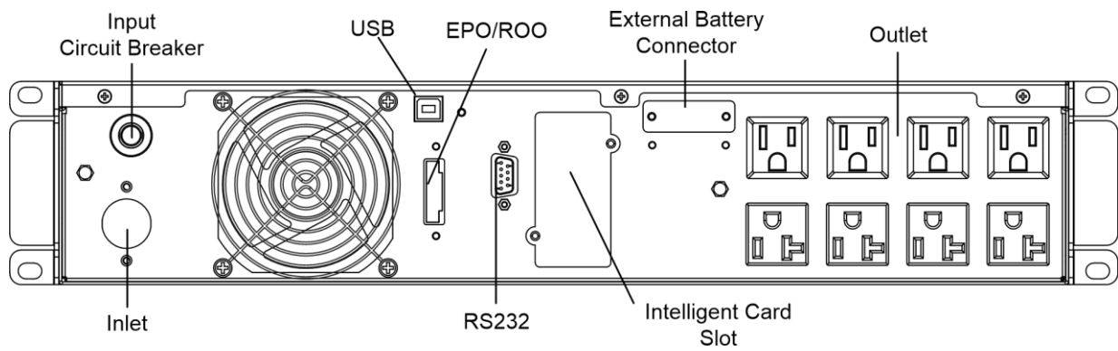
Castle-2000RM-LV 後面板視圖
