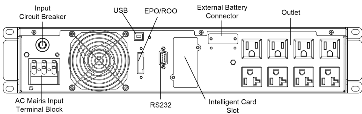
Castle Rack 2KS-LV 後面板視圖
