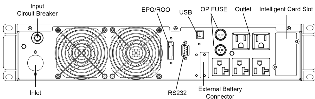
Castle-3000RM-LV 後面板視圖
