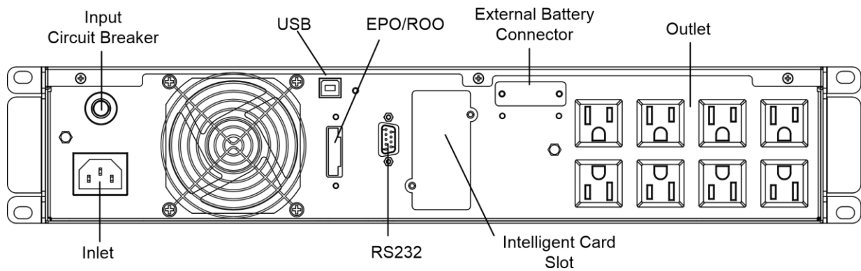
Castle-1000RM-LV 後面板視圖
