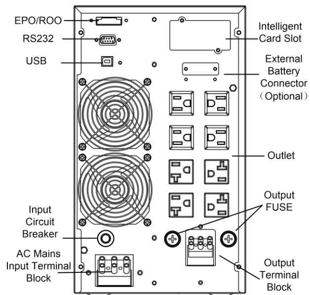
Castle Tower 3KS-LV 後面板視圖
