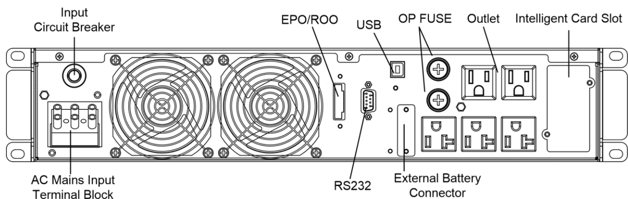
Castle Rack 3KS-LV 後面板視圖
