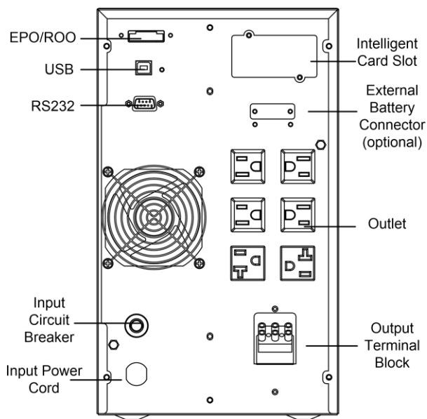
Castle Tower 2K-LV 後面板視圖
