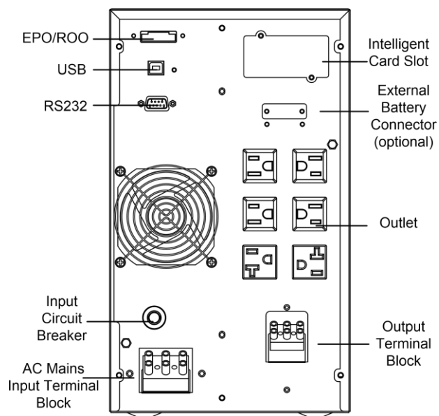
Castle Tower 2KS-LV 後面板視圖
