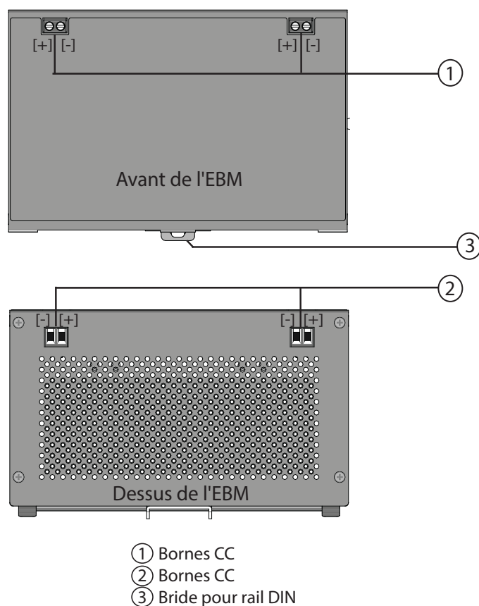
Figure 2. Caractéristiques du BPDIN24XL
