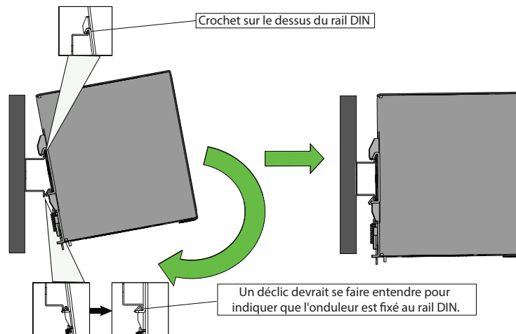
Figure 3. Montage de l'onduleur
