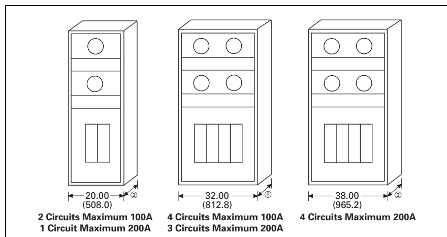
Figure 21.10-15. Fusible Switch Tenant Disconnects
