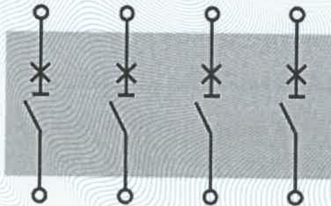
4P接线方式
