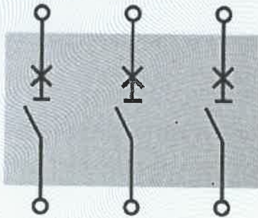
3P接线方式
