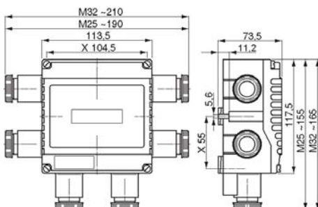
Abzweigdose GHG 791 02
