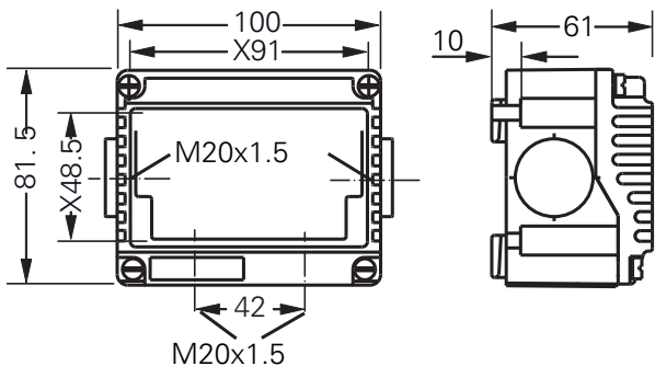
Boîte de bornes GHG 791 01
