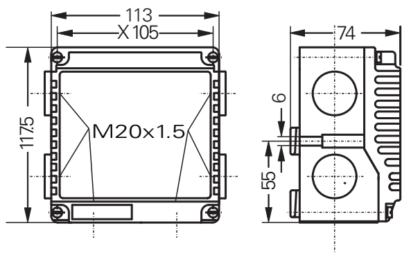
Klemmenkasten GHG 791 02
