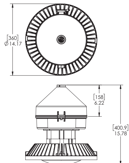
Cone pendant
