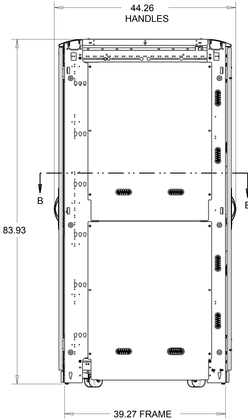
LEFT SIDE
