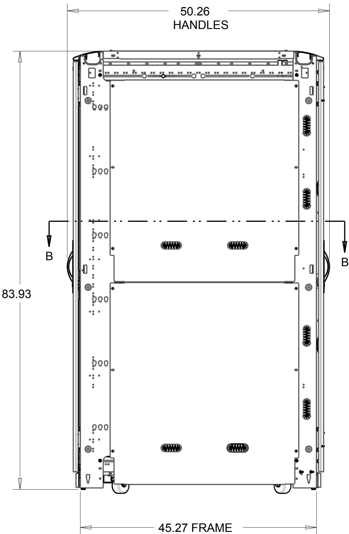
LEFT SIDE
