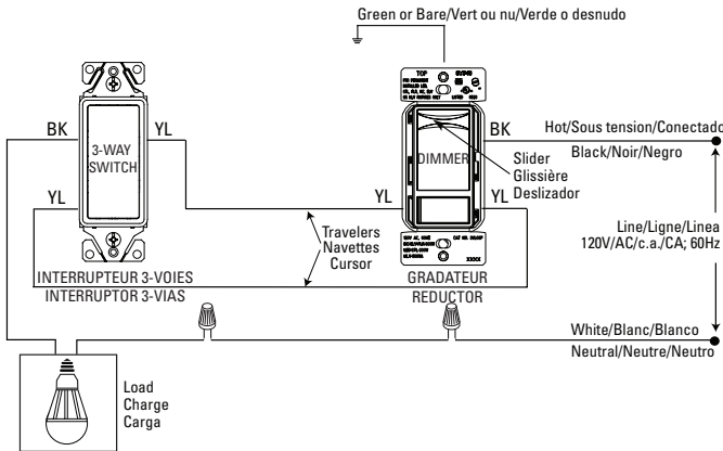
FIGURE 2: 3-WAY WIRING DIAGRAM FIGURE 2: SCHÉMA DE CÂBLAGE DE 3-VOIES FIGURA 2: DIAGRAMA DE CABLEADO DE 3-VIAS
